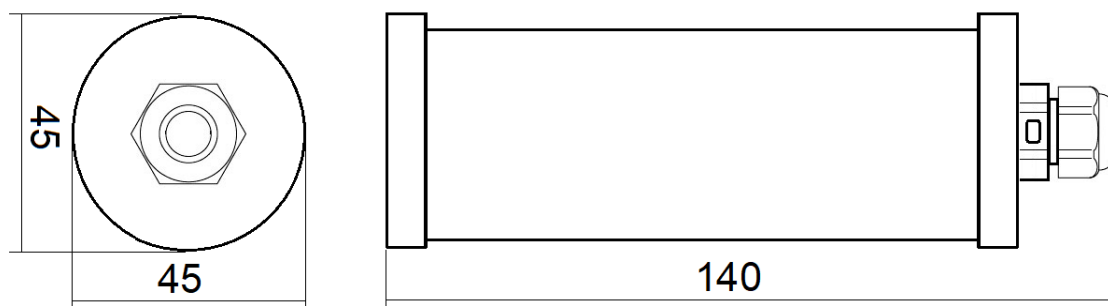
Рисунок 1 – Габаритные размеры Модуля
